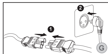
הערה: במקרה והינך צריך לחבר את ה- Innera Molla לשקע סטנדרטי, יש לרכוש כבל הזנה בנפרד אשר לא כלול כחלק מהערכה ולחברו בהתאם לאיור.
