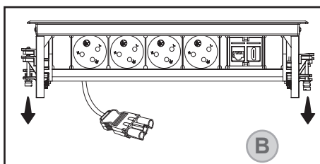
הסר/י מן ה Innera Molla את 4 אביזרי הנעילה על ידי משיכתם ודחיפתם כלפי מטה לאורך המסילות.
