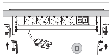
הדק/י את 4 אביזרי הנעילה על ידי החדרתם למסילות והידוקן מתחת למשטח כלפי מעלה בעזרת הברגים בחוזקה.
