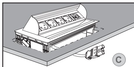
החדר/י את ה Innera Molla לתוך החור.
